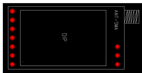
模块封装 2：DIP 插装
